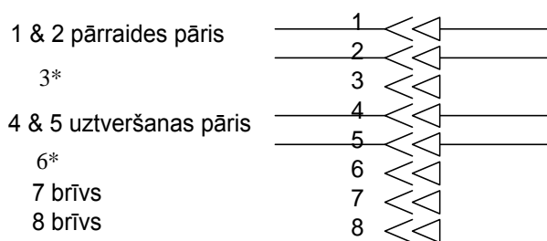
Pieslēguma shēma
